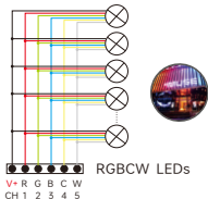
RGBCW mode
